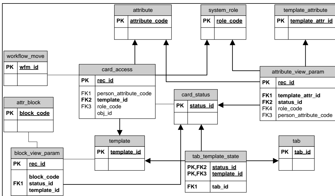
Рисунок 25 – Взаимодействие таблиц прав и состояний
