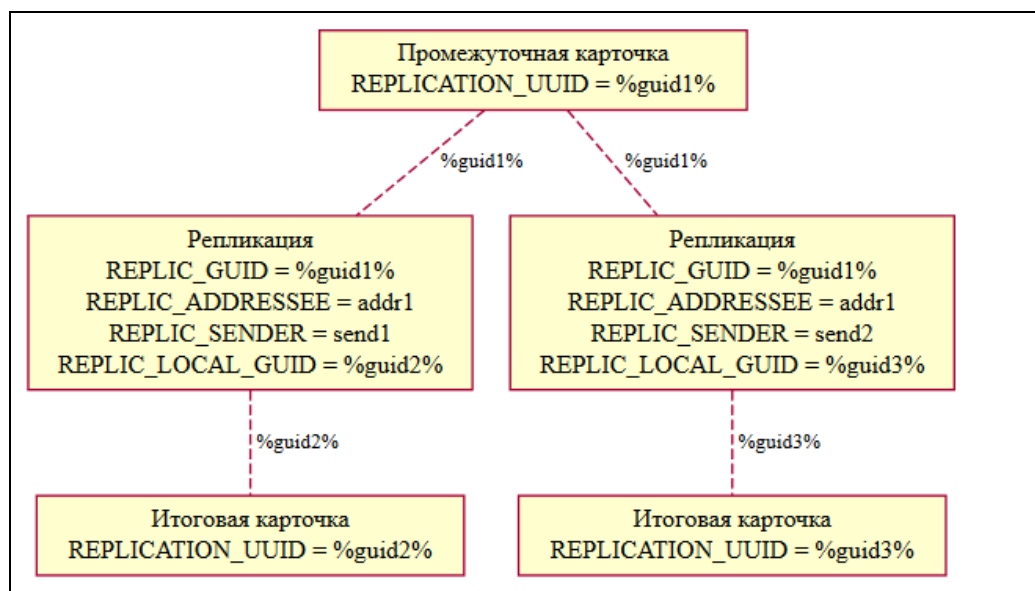
Рисунок 14 – Схема связи промежуточной и итоговой карточек
