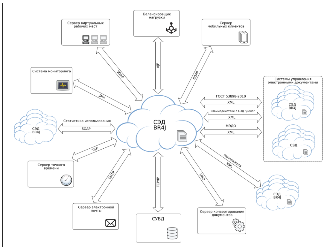
Рисунок 17 - Общая схема взаимодействия СЭД Росжелдора с внешними системами
