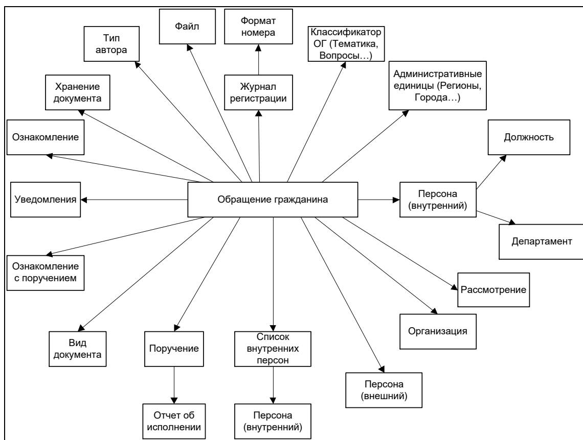
Рисунок 4 – Взаимосвязь шаблона «Обращения граждан» с шаблонами Системы
