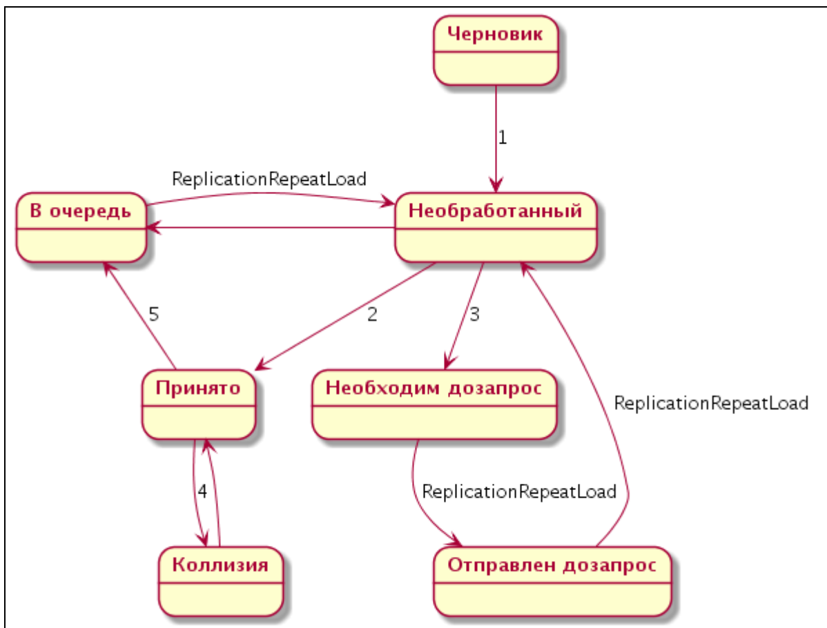
Рисунок 13 – Жизненный цикл карточек шаблона «Репликация» для механизма загрузки данных
