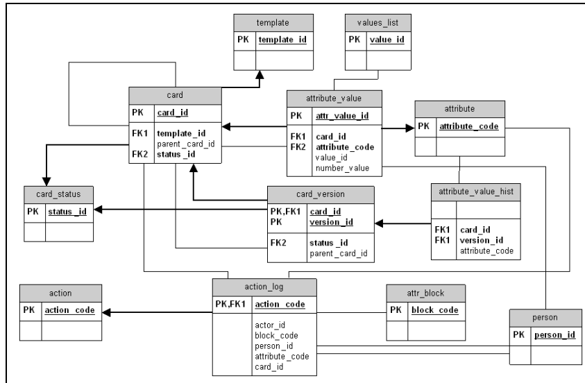
Рисунок 24 – Взаимодействие таблиц значений и истории
