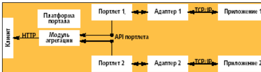
Рисунок 15 - Обобщенная схема «традиционной» интеграции
