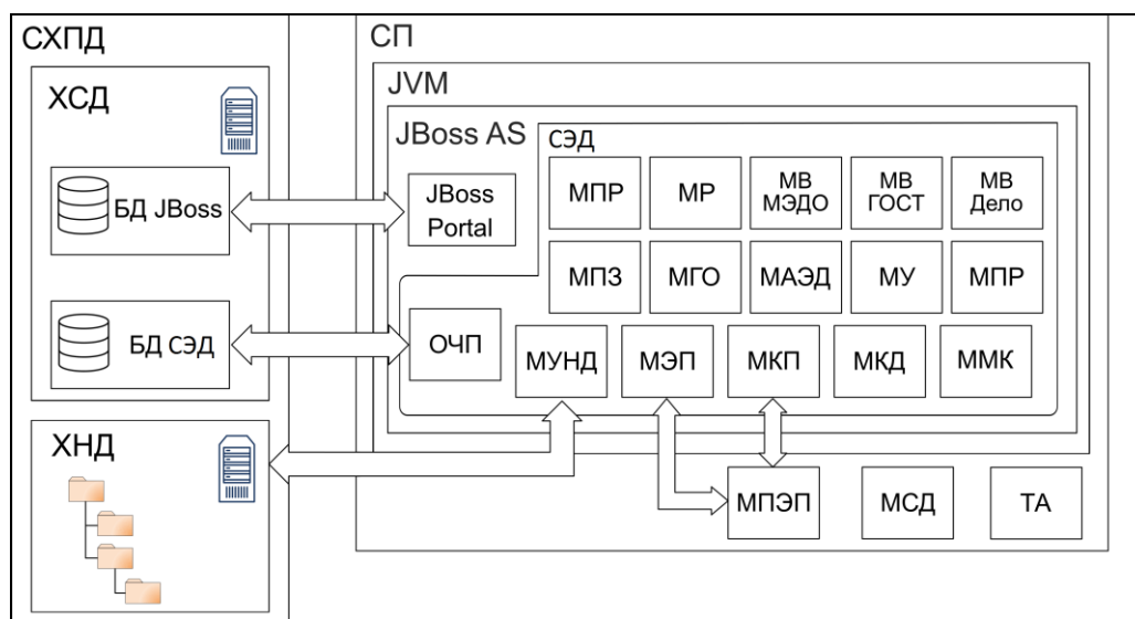
Рисунок 6 – Схема модулей системы
