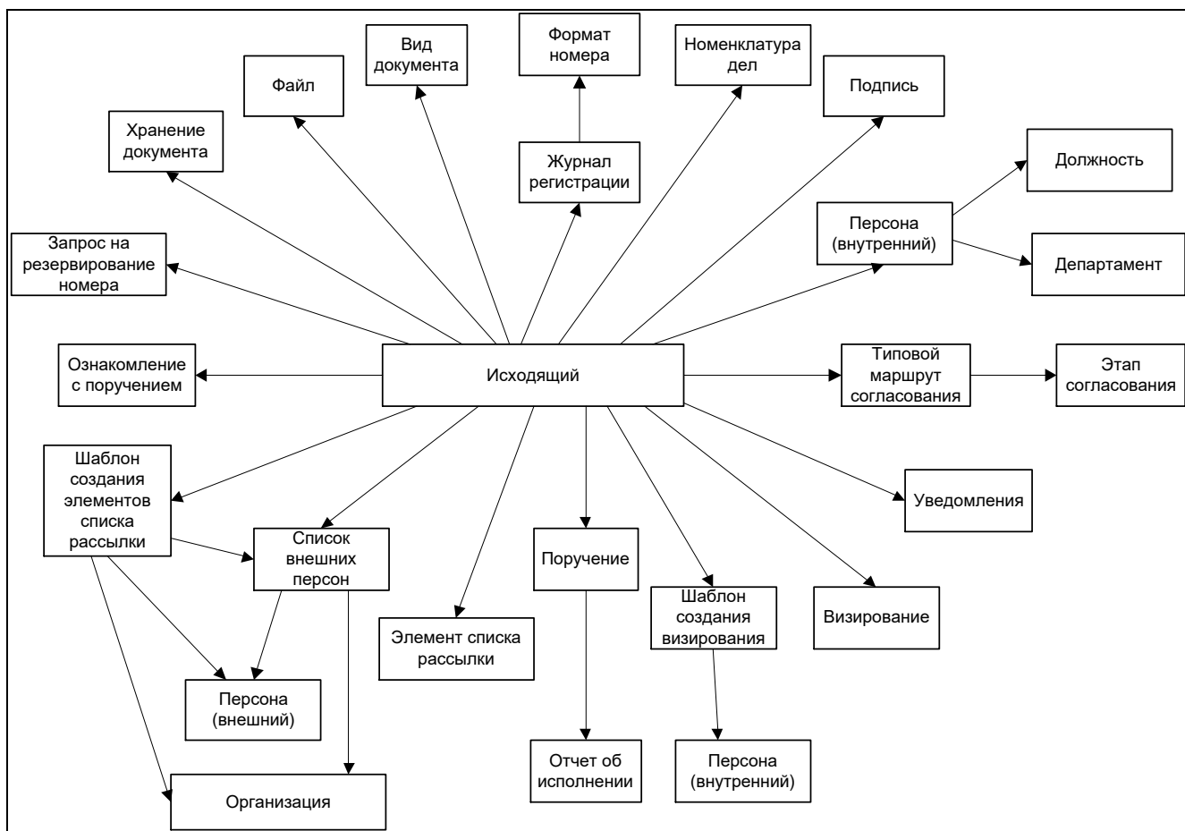
Рисунок 2 – Взаимосвязь шаблона «Исходящий» с шаблонами Системы
