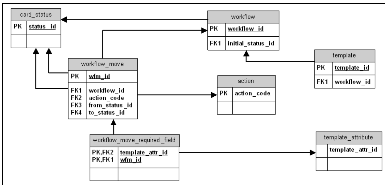
Рисунок 22 – Взаимодействие таблиц ЖЦ
