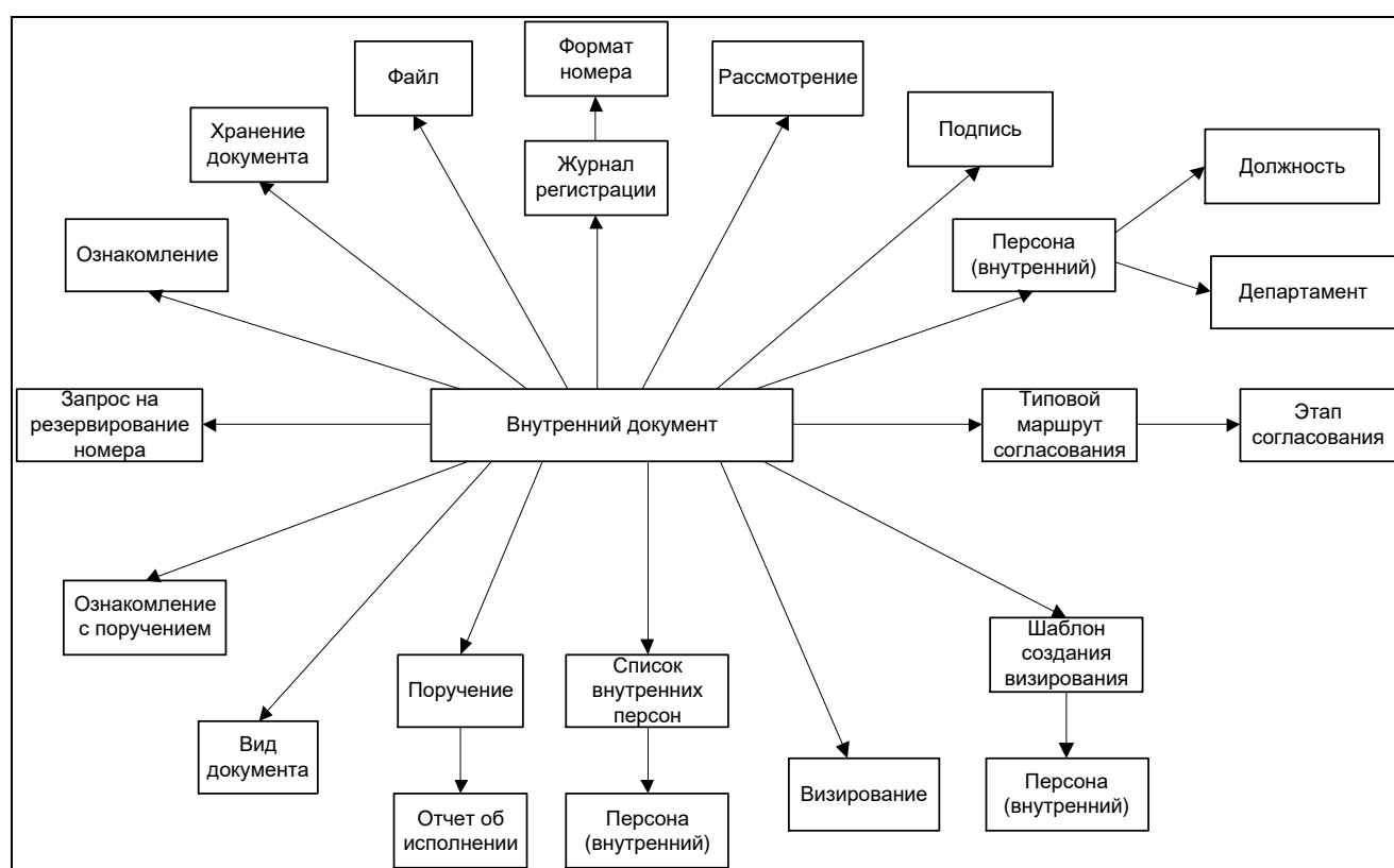
Рисунок 3 – Взаимосвязь шаблона «Внутренний» с шаблонами Системы
