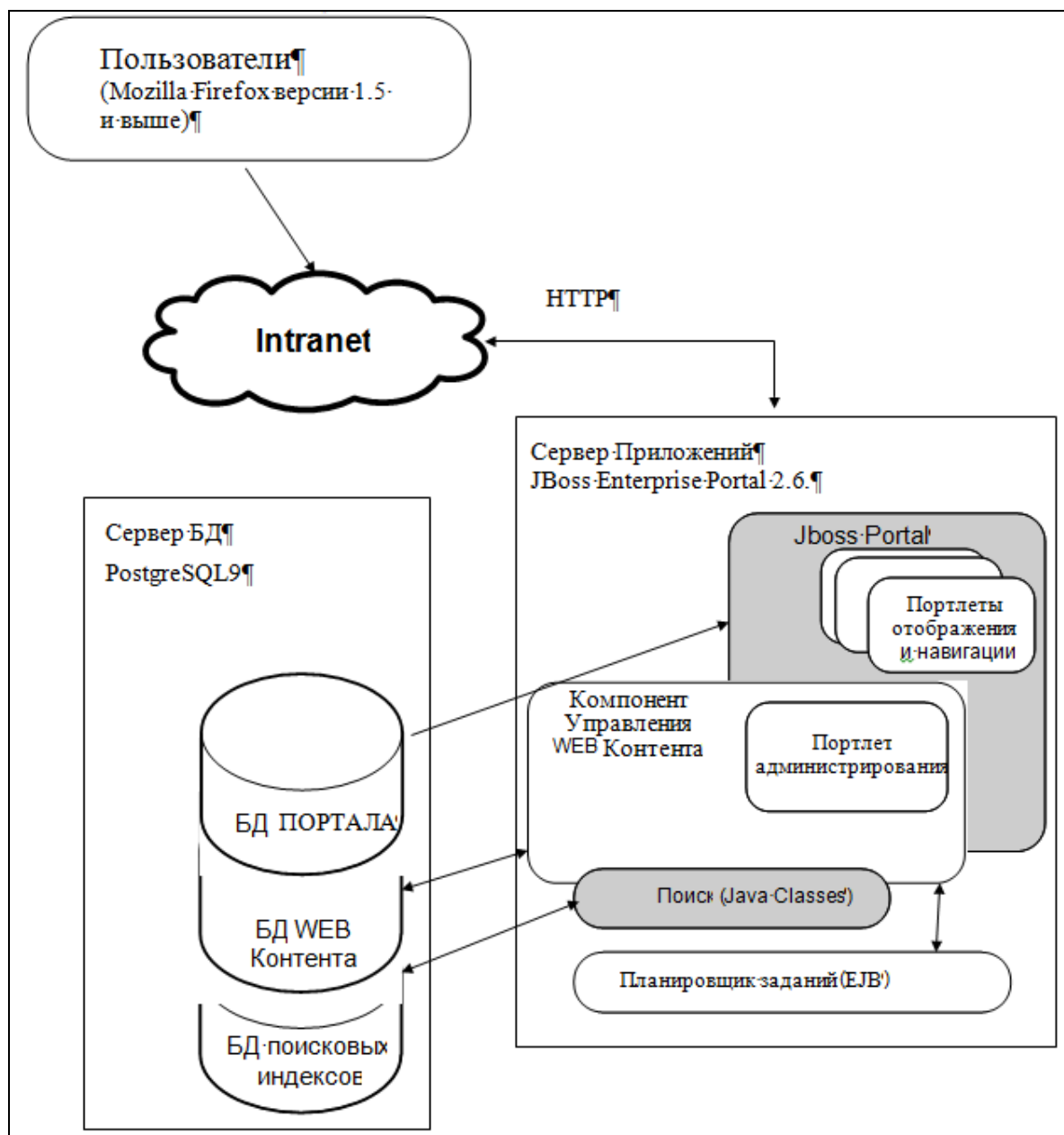
Рисунок 19 - Схема взаимодействия компонентов системы
