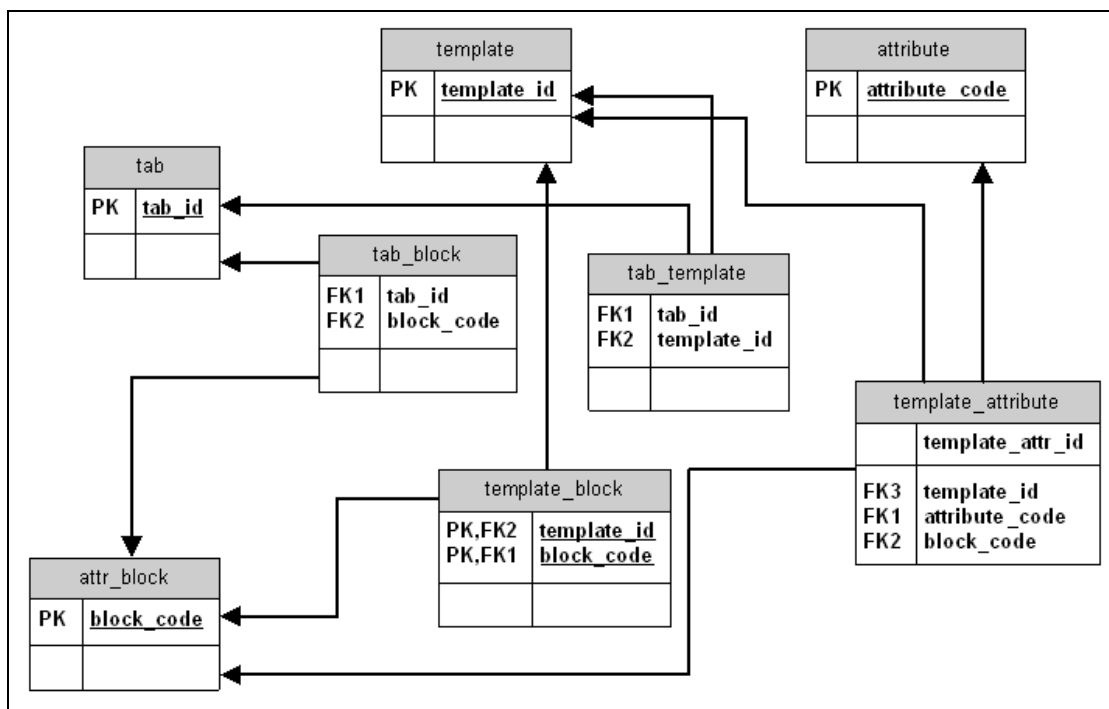
Рисунок 20 – Взаимодействие таблиц структуры
