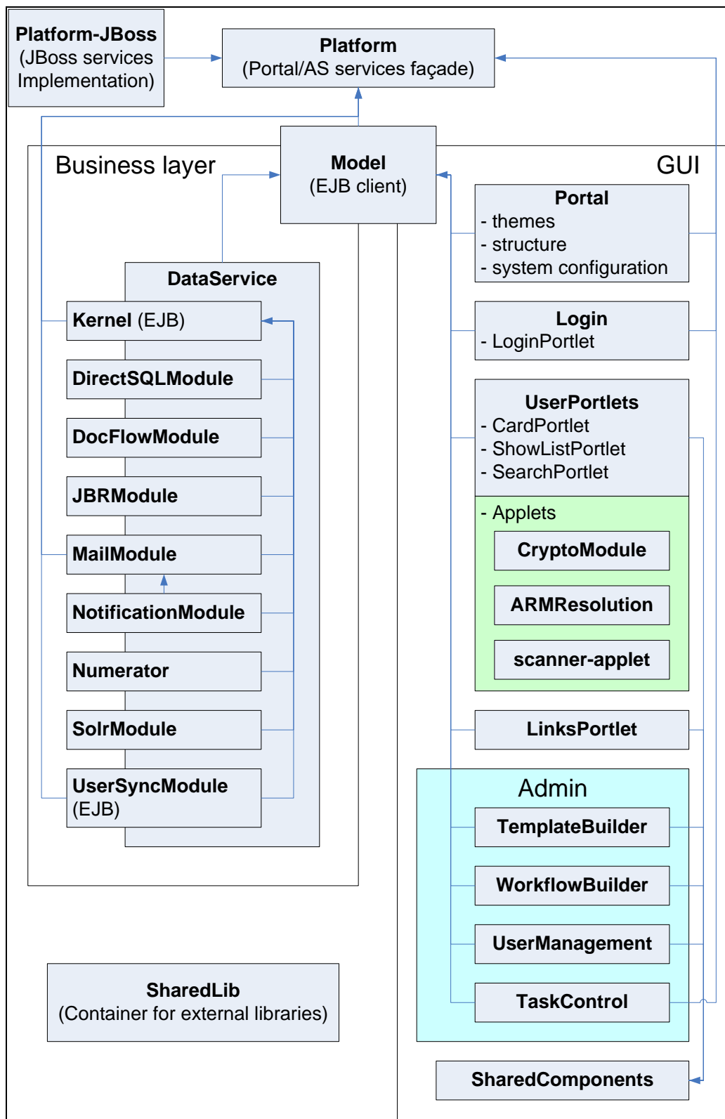
Рисунок 27 – Схема взаимосвязи проектов
