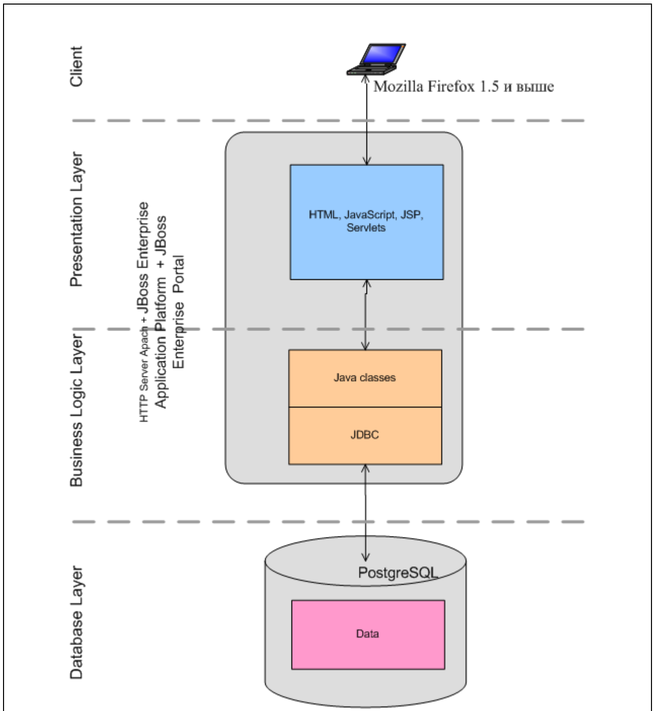
Рисунок 18 - Трехуровневая модель архитектуры системы
