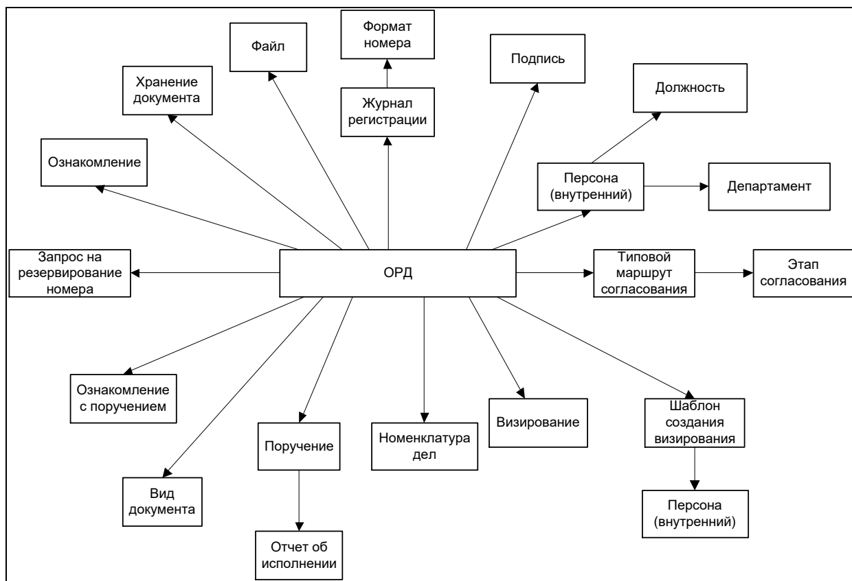
Рисунок 5 – Взаимосвязь шаблона «Обращения граждан» с шаблонами Системы
