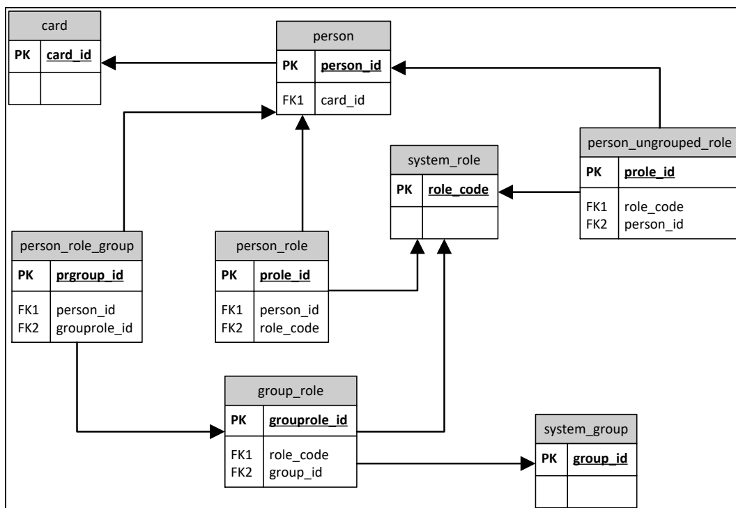
Рисунок 23 – Взаимодействие таблиц пользователей и ролей
